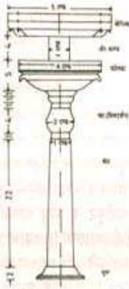
आकृती ३ खांबाचे अवयव
