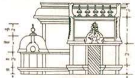
आकृती ६ सान्तरप्रस्तर कोष्ठ
