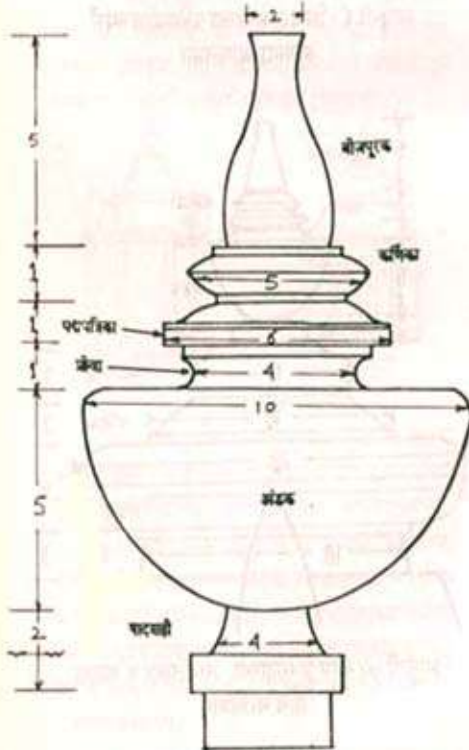
आकृती ८ : कळसाचे धरविभाग
