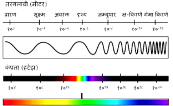
विद्युत चुंबकीय वर्णपट
